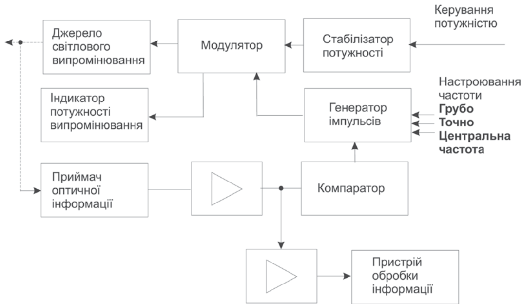
Рис. 2. Структурна схема лазерного апарату «Промінь-12»
