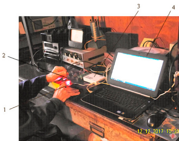
Рис. 8. Экспериментальная установка: 1 — светодиод, 2 — фотодиод, 3 — аналого-цифровой преобразователь, 4 — компьютер
